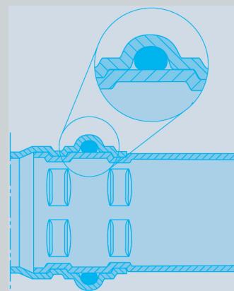
Przekrój zaprasowanej złączki Viega.
